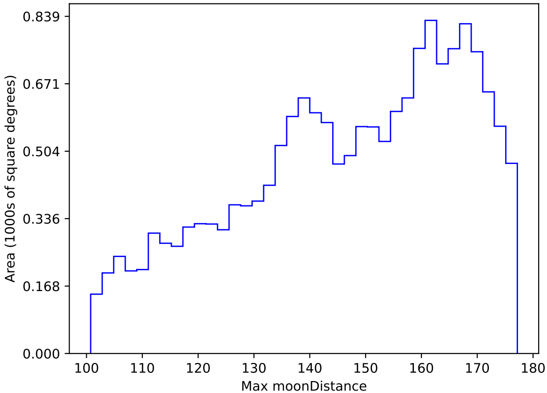
too_elab_r256_d2_ugrizy_v3.4_10yrs WFD y band: Max moonDistance
