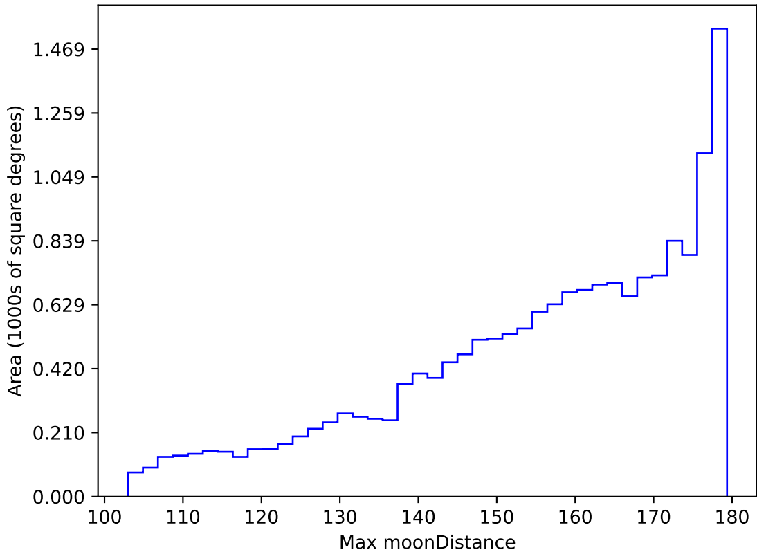
too_elab_r256_d2_ugrizy_v3.4_10yrs WFD r band: Max moonDistance
