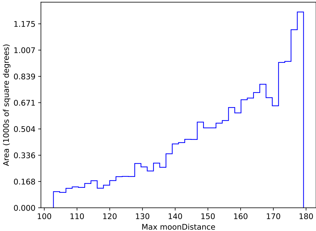
too_elab_r256_d2_ugrizy_v3.4_10yrs WFD i band: Max moonDistance
