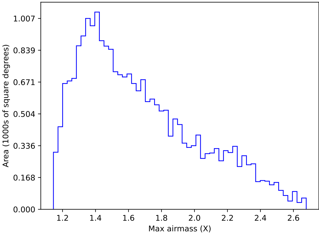
too_elab_r256_d2_ugrizy_v3.4_10yrs Yr 1 y band: Max airmass
