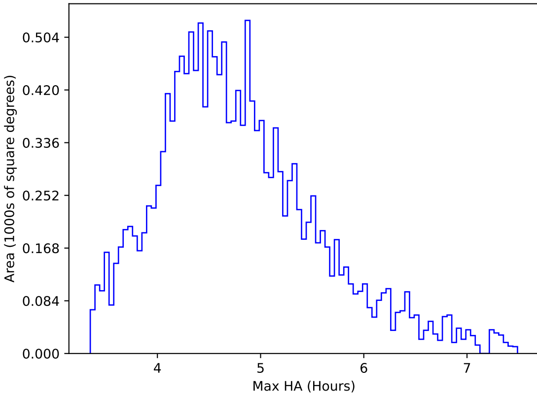
too_elab_r256_d2_ugrizy_v3.4_10yrs WFD y band: Max HA
