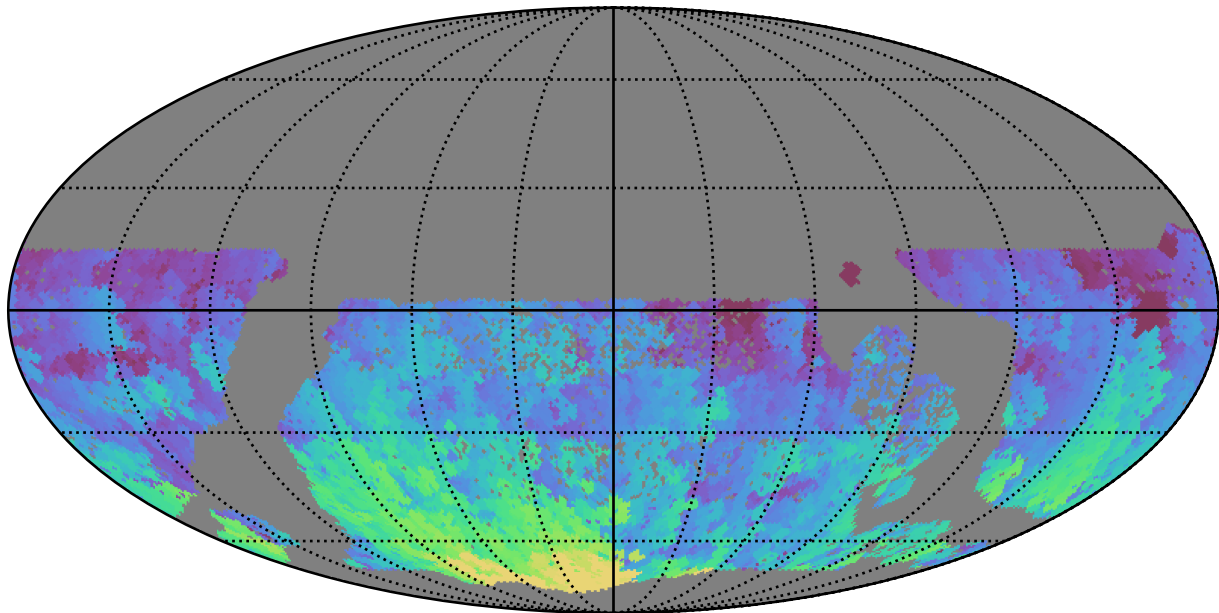
too_elab_r256_d2_ugrizy_v3.4_10yrs WFD u band: Max HA
