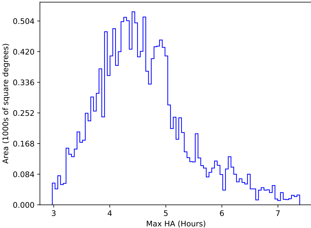
too_elab_r256_d2_ugrizy_v3.4_10yrs WFD r band: Max HA
