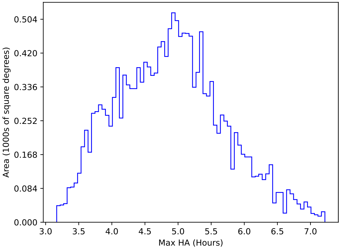
too_elab_r256_d2_ugrizy_v3.4_10yrs WFD i band: Max HA
