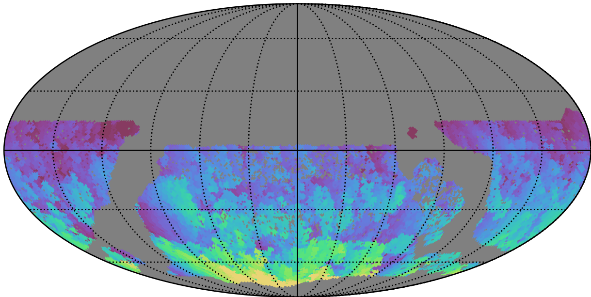
too_elab_r256_d2_ugrizy_v3.4_10yrs WFD g band: Max HA
