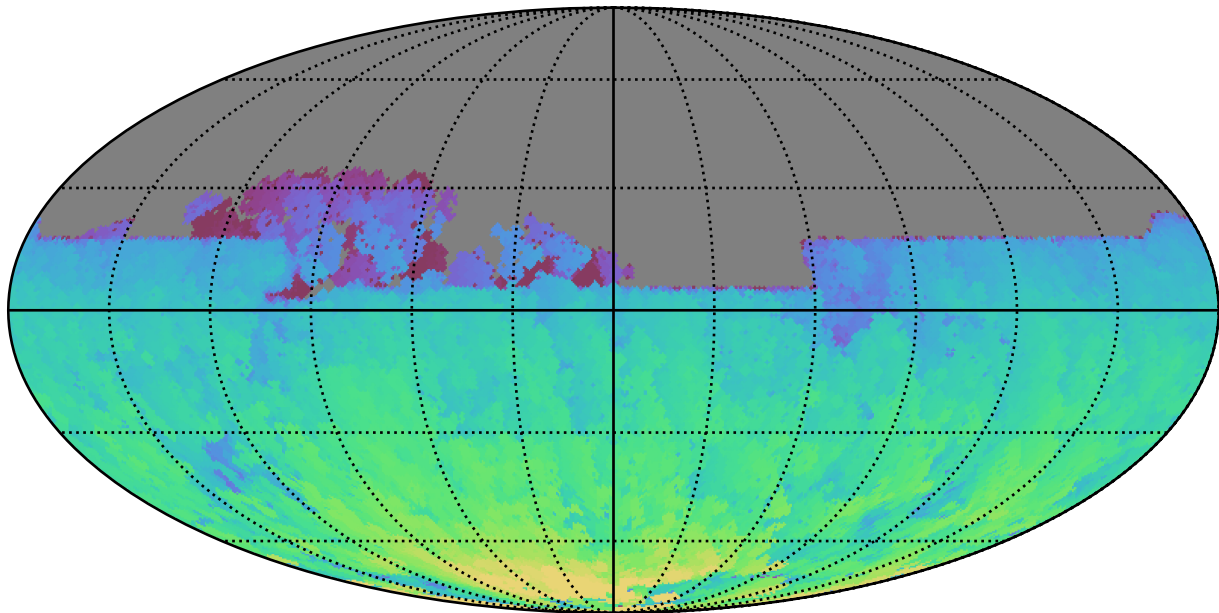
too_elab_r256_d2_ugrizy_v3.4_10yrs All sky y band: Max HA
