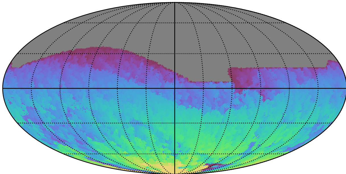
too_elab_r256_d2_ugrizy_v3.4_10yrs All sky i band: Max HA
