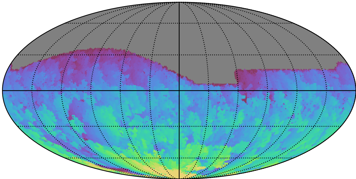
too_elab_r256_d2_ugrizy_v3.4_10yrs All sky g band: Max HA
