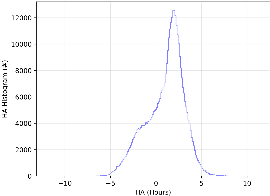
too_elab_r256_d2_ugrizy_v3.4_10yrs WFD y band: HA Histogram
