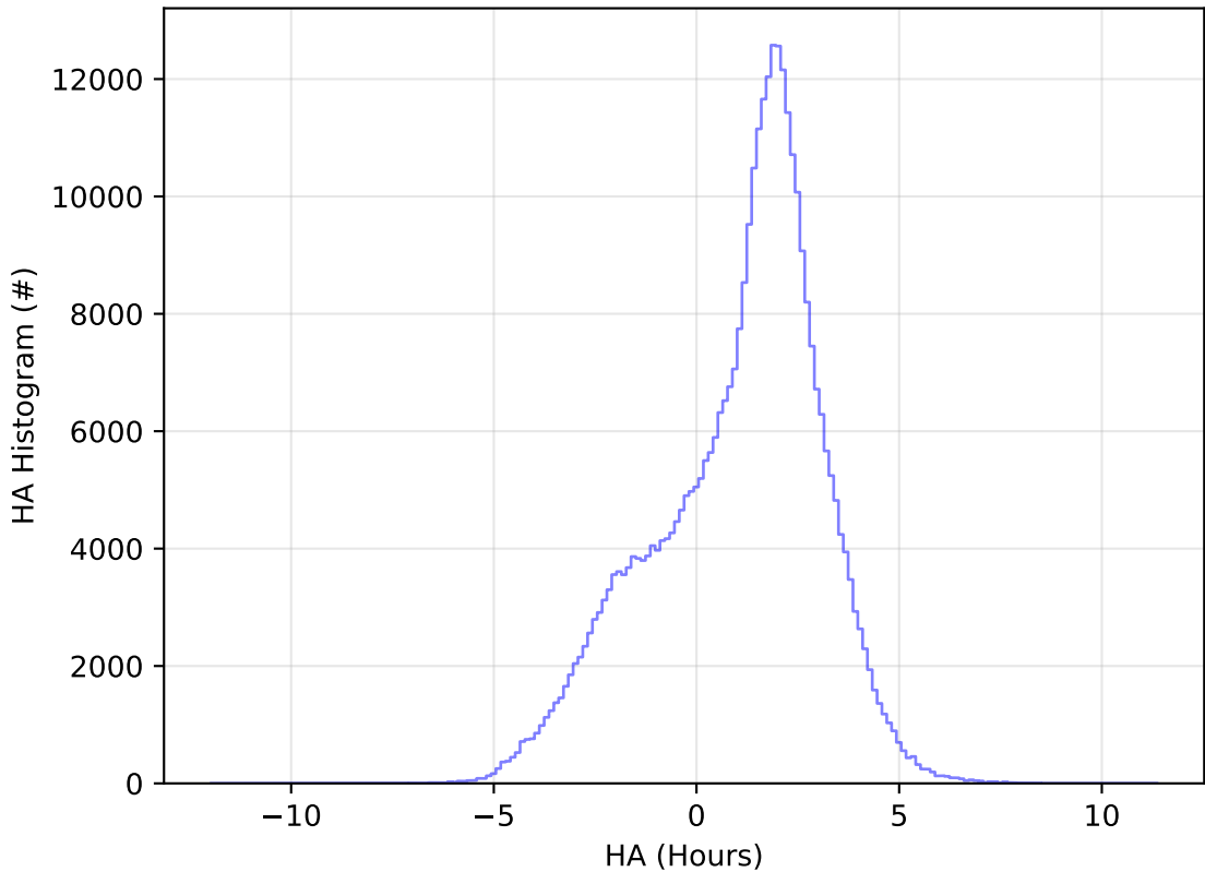
too_elab_r256_d2_ugrizy_v3.4_10yrs All sky y band: HA Histogram
