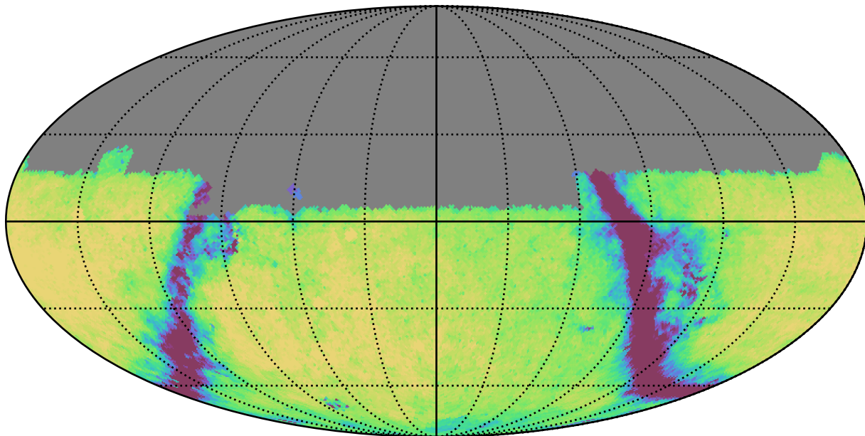
too_elab_r256_d2_ugrizy_v3.4_10yrs Yr 1 u band: Exgal_CoaddM5
