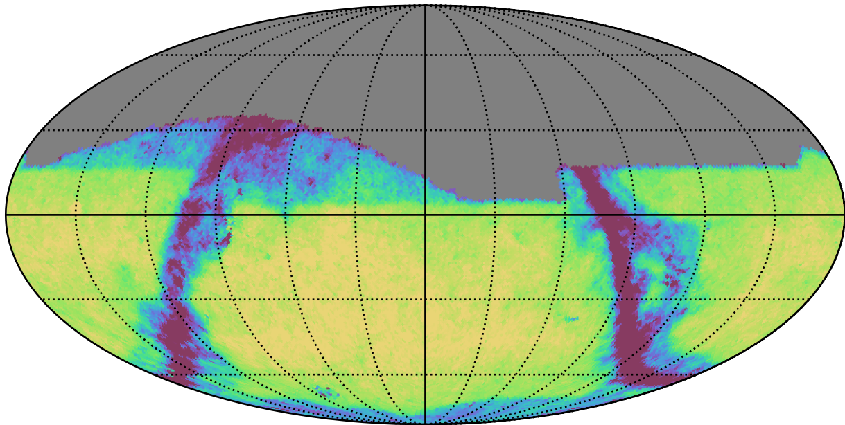
too_elab_r256_d2_ugrizy_v3.4_10yrs Yr 1 i band: Exgal_CoaddM5
