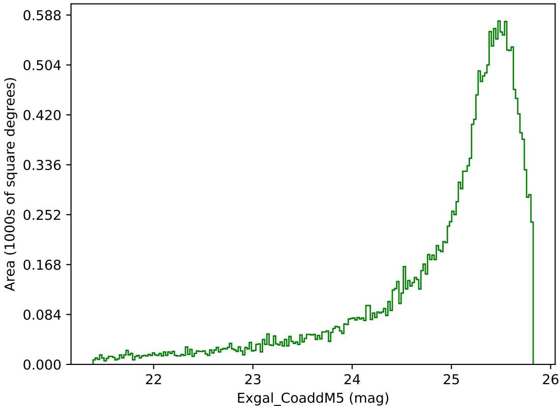
too_elab_r256_d2_ugrizy_v3.4_10yrs Yr 1 g band: Exgal_CoaddM5
