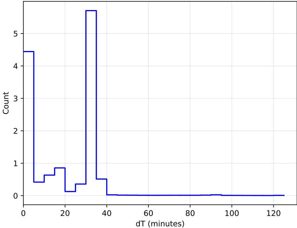
too_elab_r256_d2_ugrizy_v3.4_10yrs All sky: DeltaT Histogram 1e6
