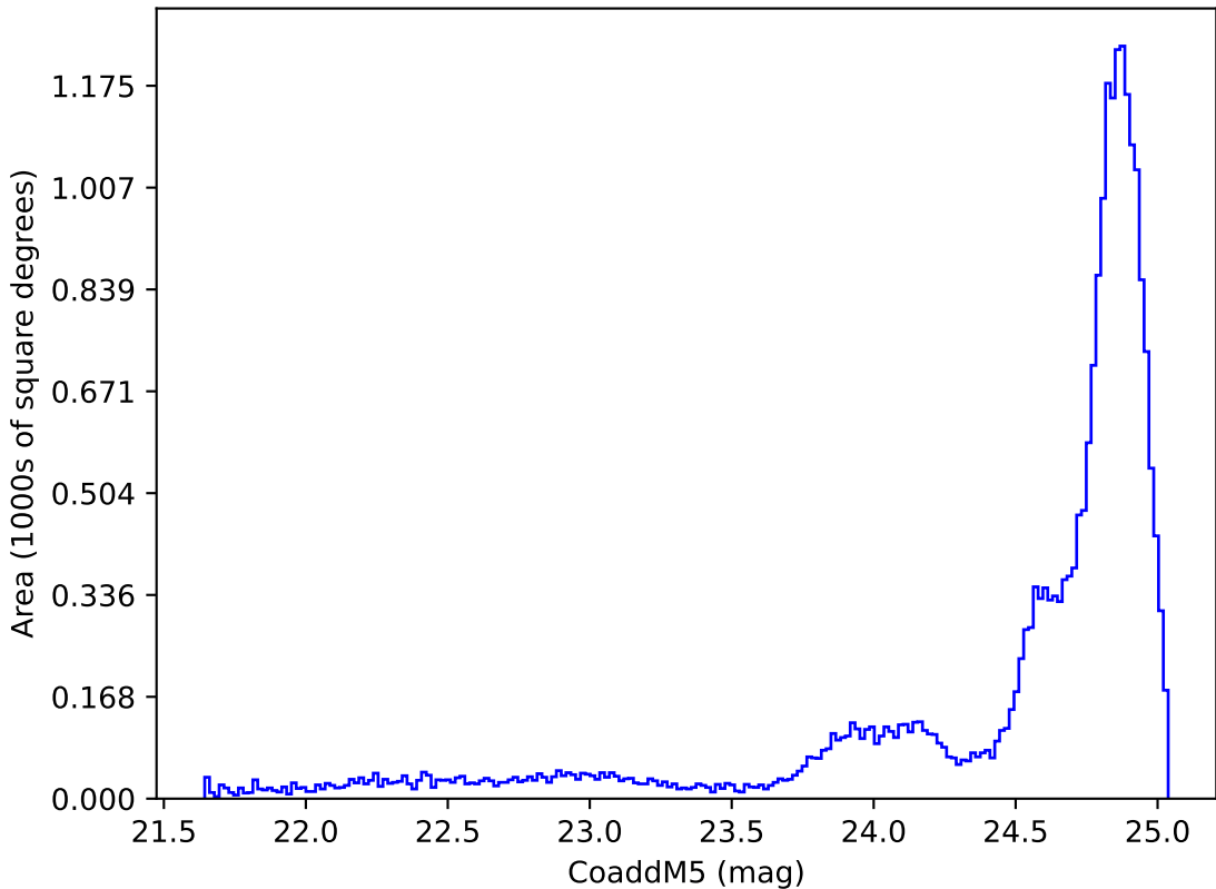
too_elab_r256_d2_ugrizy_v3.4_10yrs All sky y band: CoaddM5
