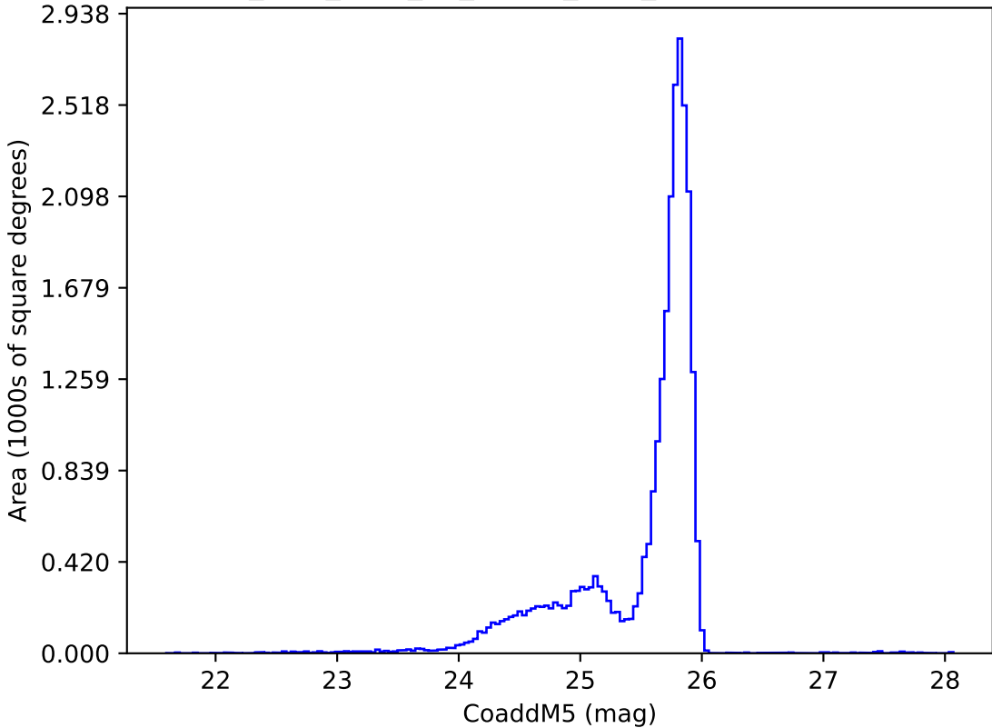
too_elab_r256_d2_ugrizy_v3.4_10yrs z: CoaddM5
