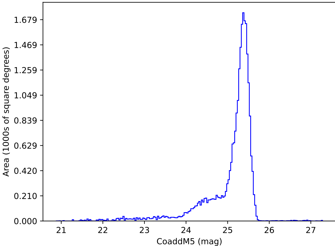
too_elab_r256_d2_ugrizy_v3.4_10yrs u: CoaddM5
