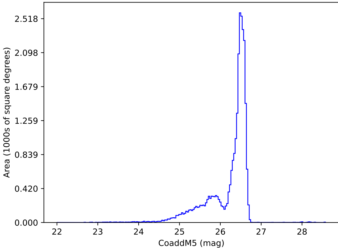
too_elab_r256_d2_ugrizy_v3.4_10yrs i: CoaddM5
