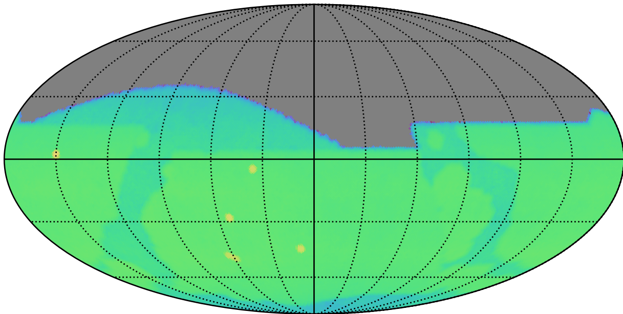
too_elab_r256_d2_ugrizy_v3.4_10yrs : CoaddM5
