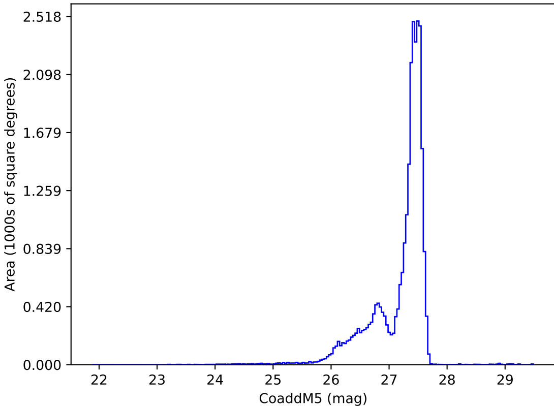
too_elab_r256_d2_ugrizy_v3.4_10yrs : CoaddM5
