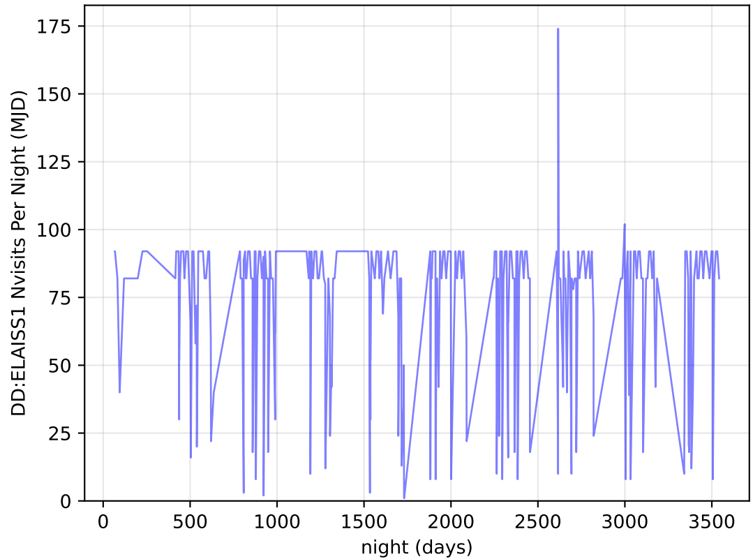
too_elab_r256_d2_ugrizy_v3.4_10yrs all bands: DD:ELAISS1 Nvisits Per Night
