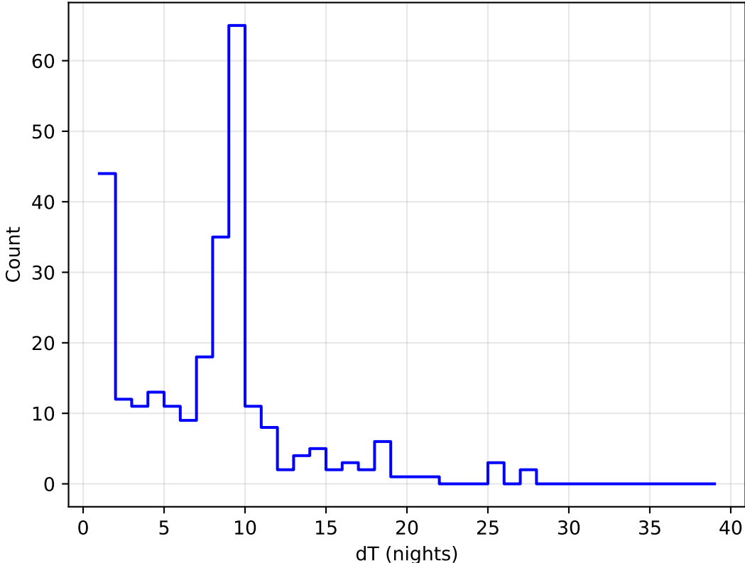
too_elab_r256_d2_ugrizy_v3.4_10yrs all bands: DD:ELAISS1 Delta Nights Histogram
