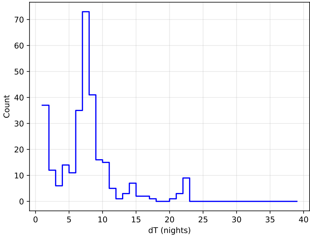
too_elab_r256_d2_ugrizy_v3.4_10yrs all bands: DD:EDFS Delta Nights Histogram
