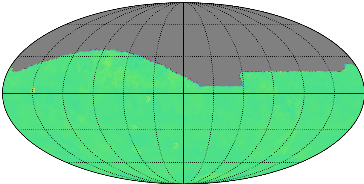
too_elab_r256_d2_gz_v3.4_10yrs i: Kuiper rotTelPos
