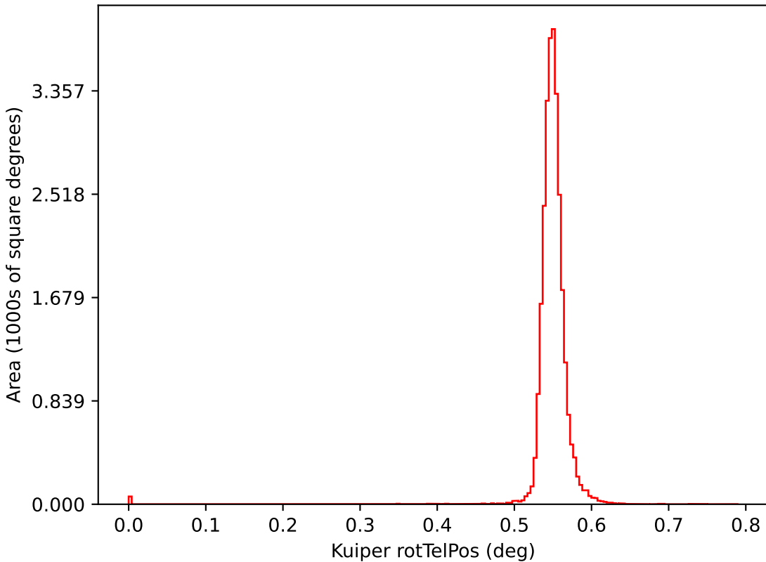
too_elab_r256_d2_gz_v3.4_10yrs i: Kuiper rotTelPos
