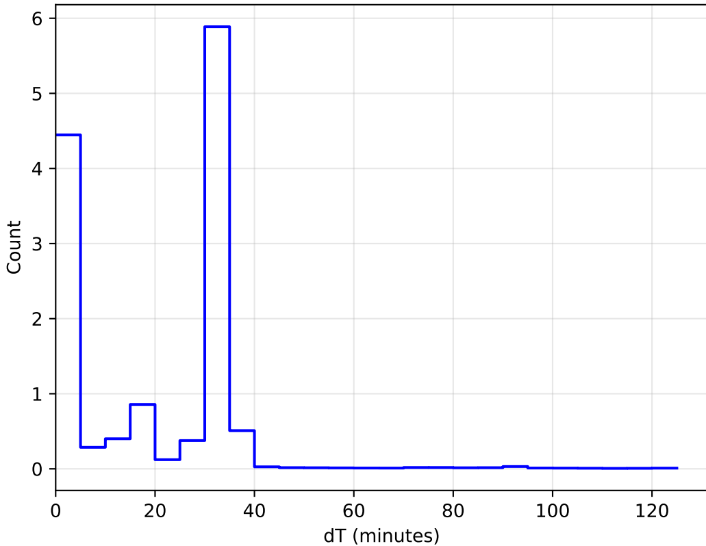
too_elab_r256_d2_gz_v3.4_10yrs All sky: DeltaT Histogram 1e6
