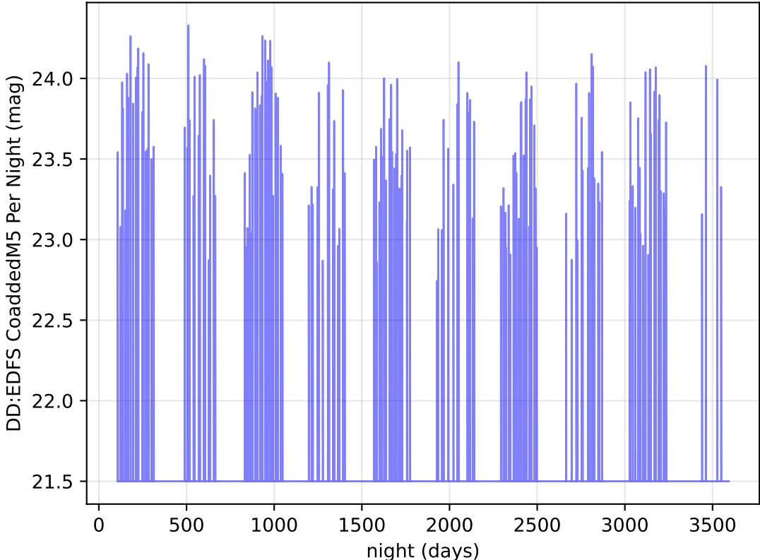
too_elab_r256_d2_gz_v3.4_10yrs y band: DD:EDFS CoaddedM5 Per Night
