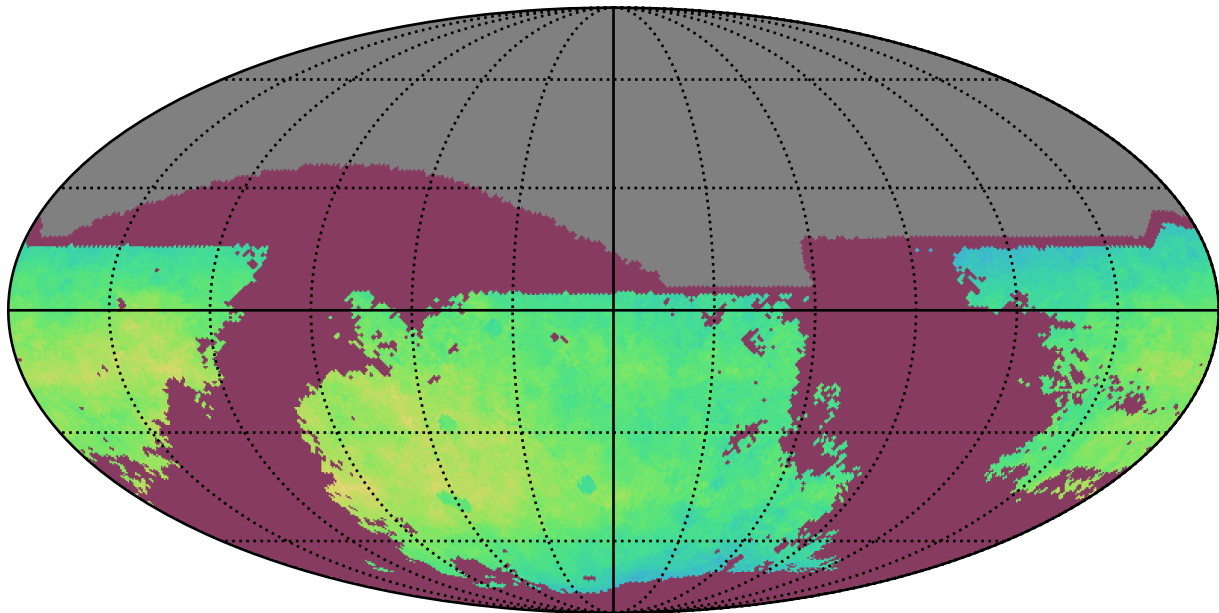
too_elab_r256_d2_griz_v3.4_10yrs i: NgalScale
