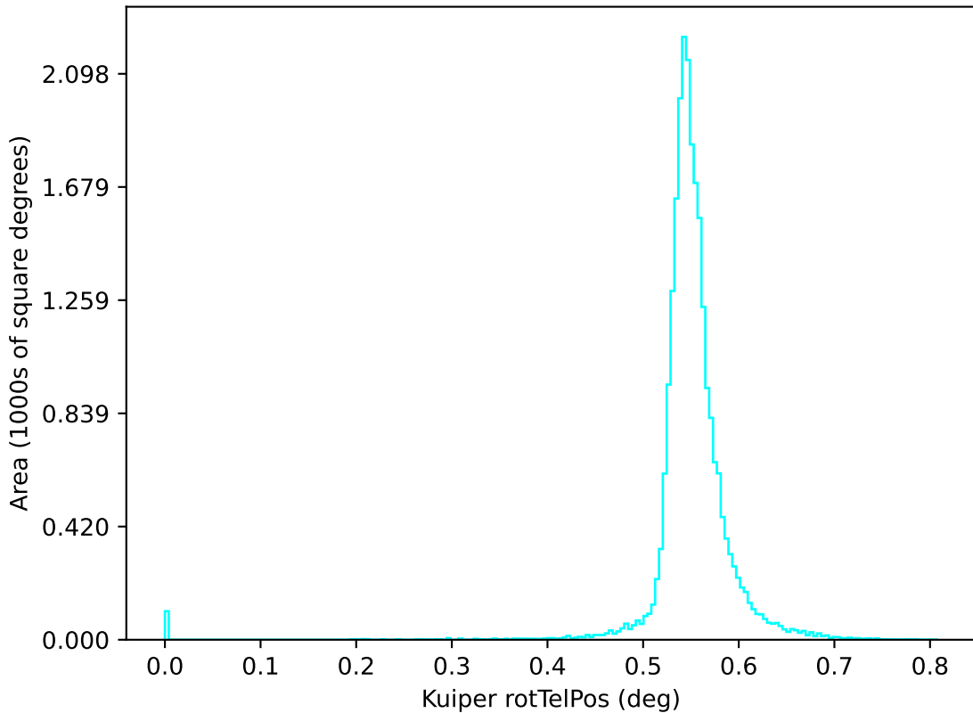
too_elab_r256_d2_griz_v3.4_10yrs u: Kuiper rotTelPos
