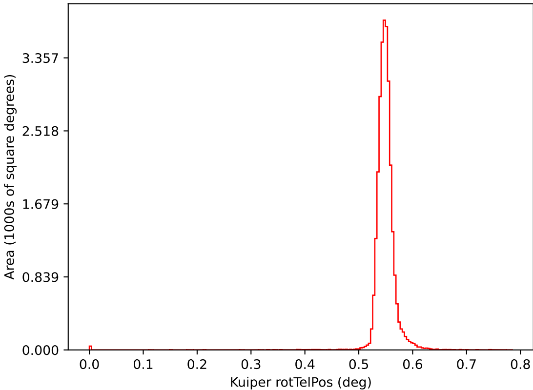
too_elab_r256_d2_griz_v3.4_10yrs i: Kuiper rotTelPos
