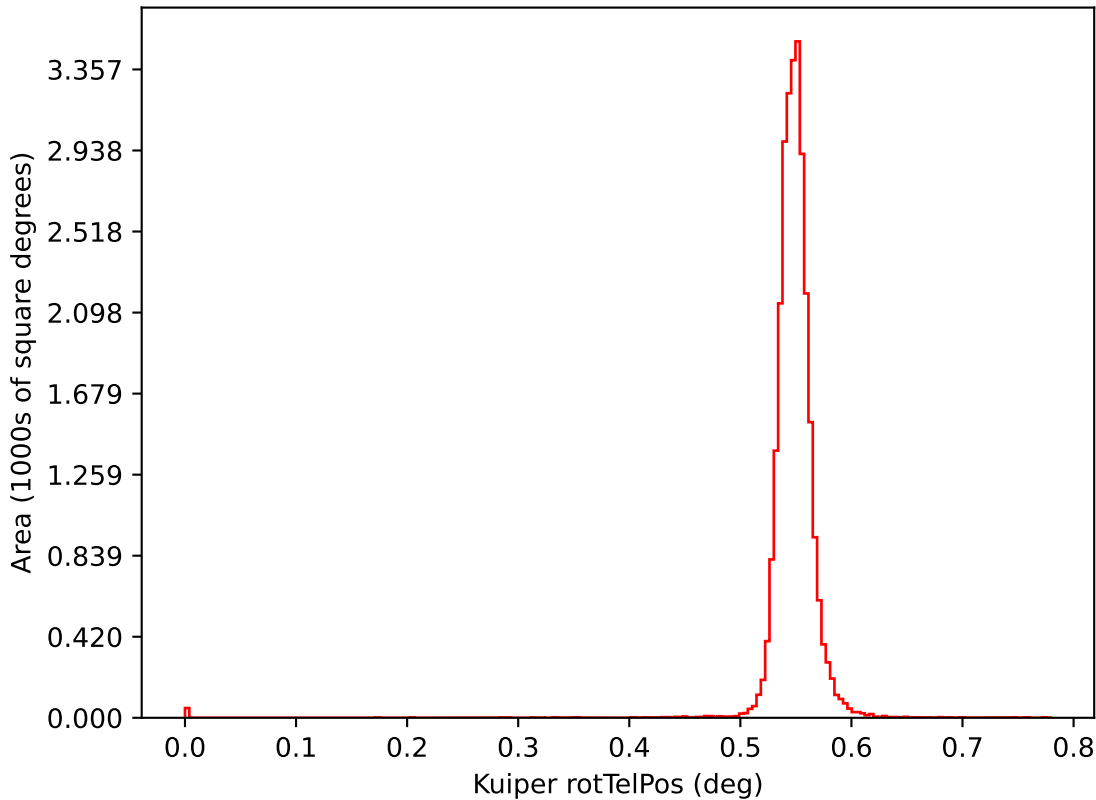
too_elab_r256_d2_giz_v3.4_10yrs i: Kuiper rotTelPos
