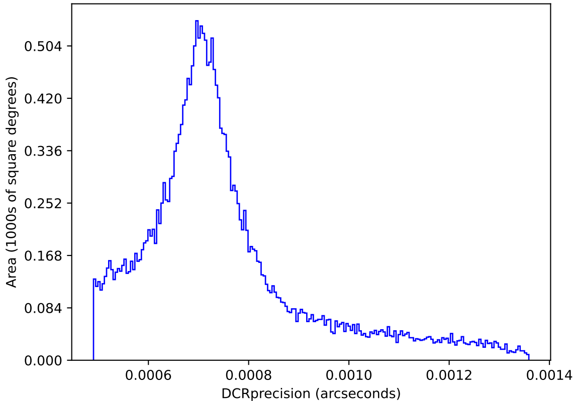
too_elab_r256_d2_giz_v3.4_10yrs : DCRprecision
