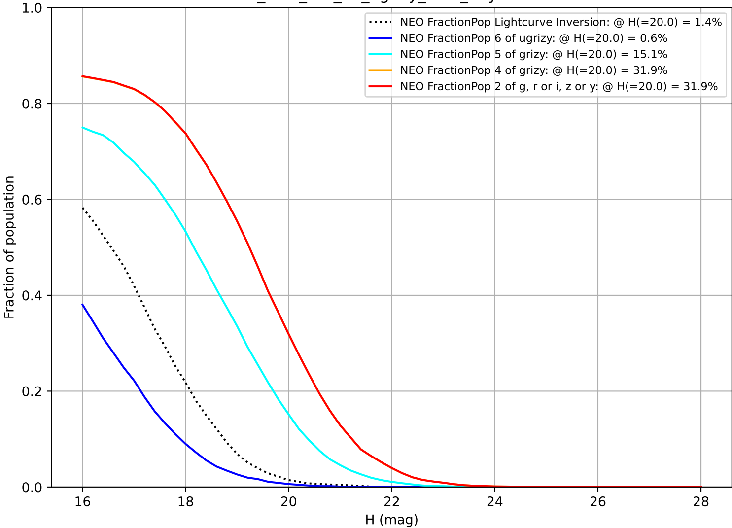
too_elab_r16_d3_ugrizy_v3.4_10yrs NEO
