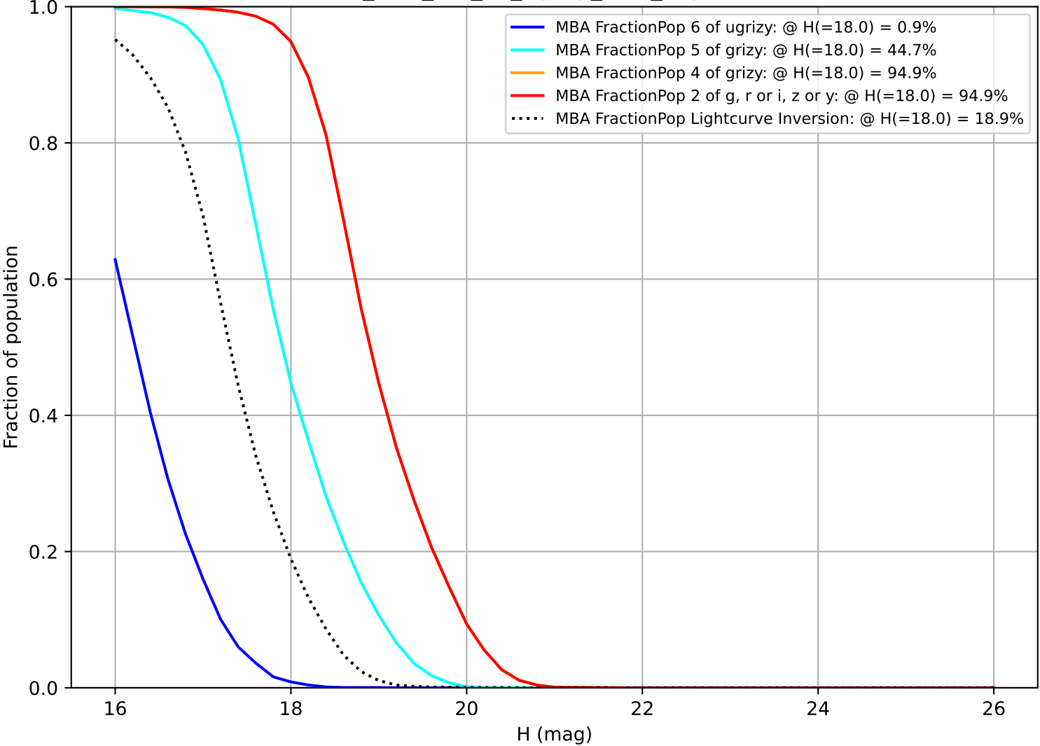
too_elab_r16_d3_ugrizy_v3.4_10yrs MBA
