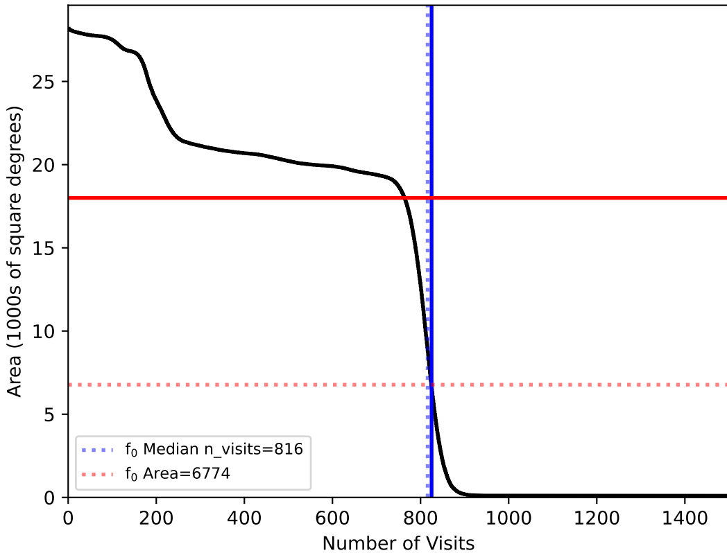
too_elab_r16_d3_ugrizy_v3.4_10yrs : f0
