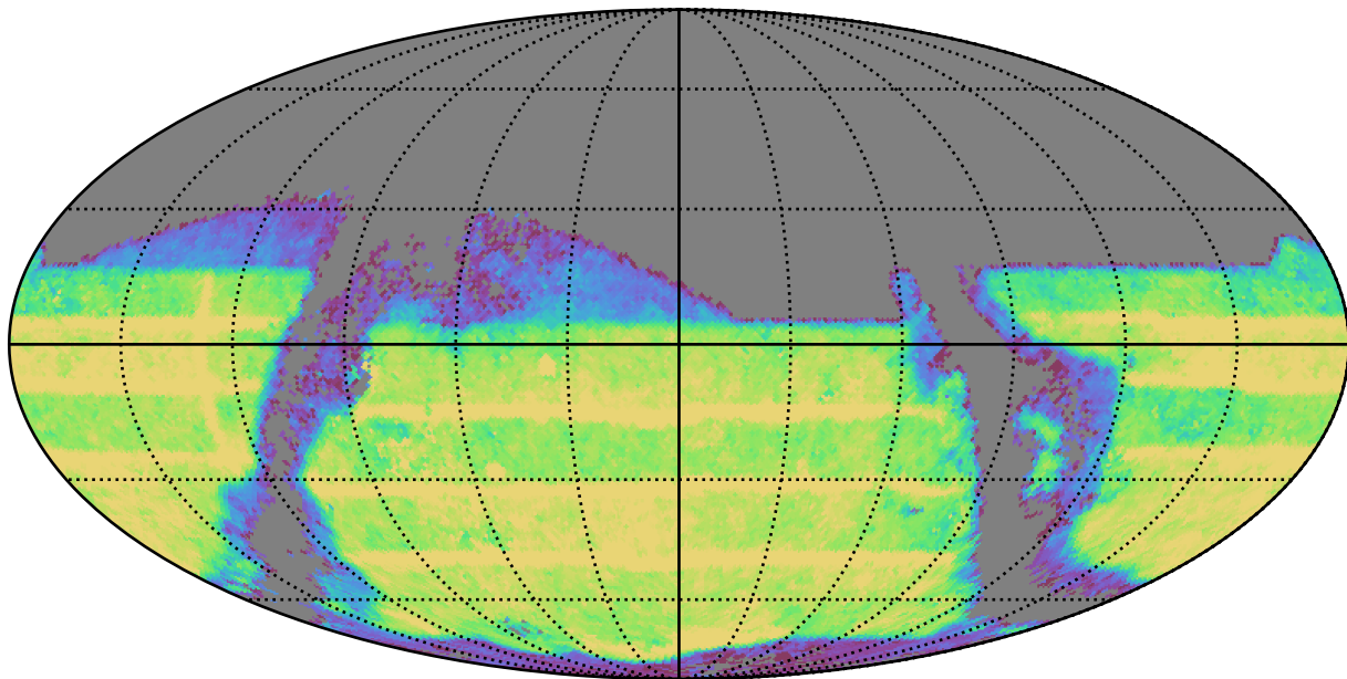
too_elab_r16_d3_ugrizy_v3.4_10yrs : TDC_rate
