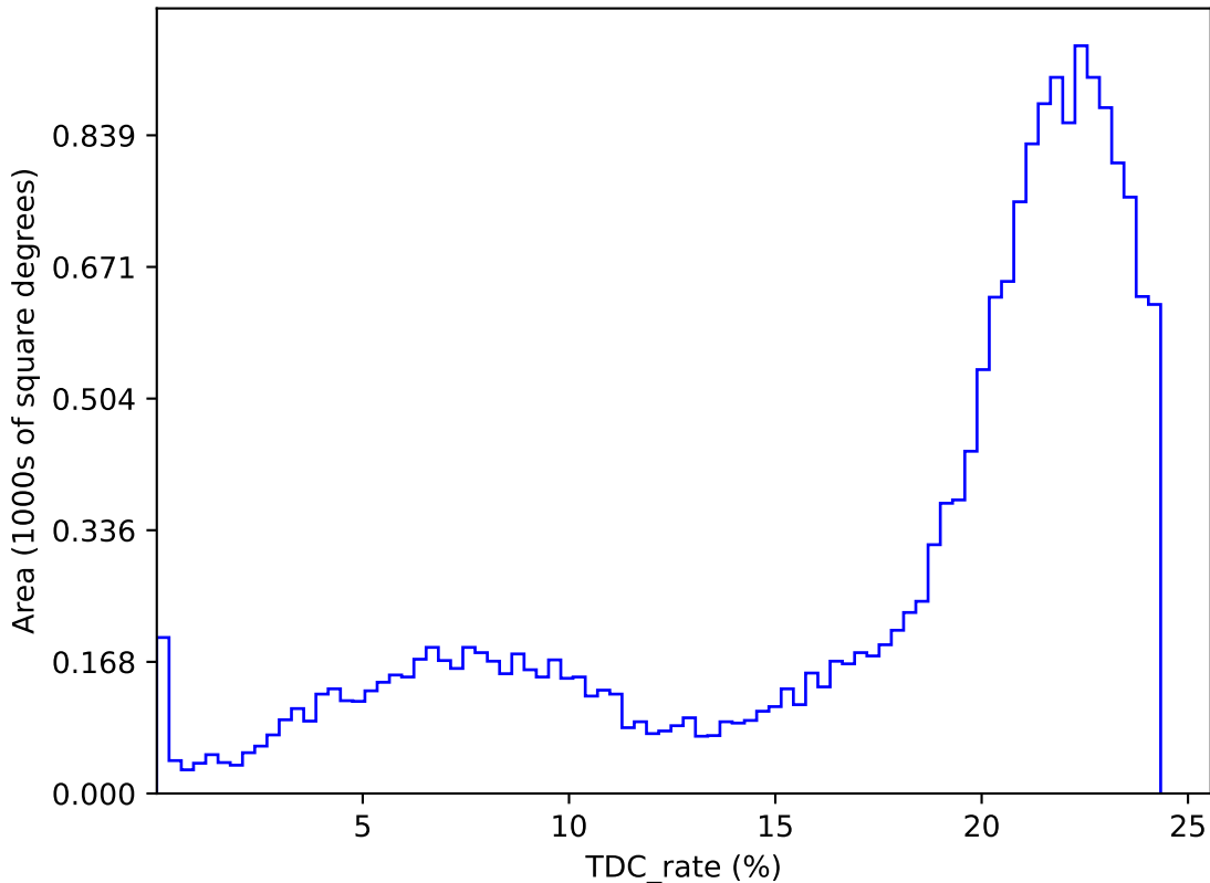
too_elab_r16_d3_ugrizy_v3.4_10yrs : TDC_rate
