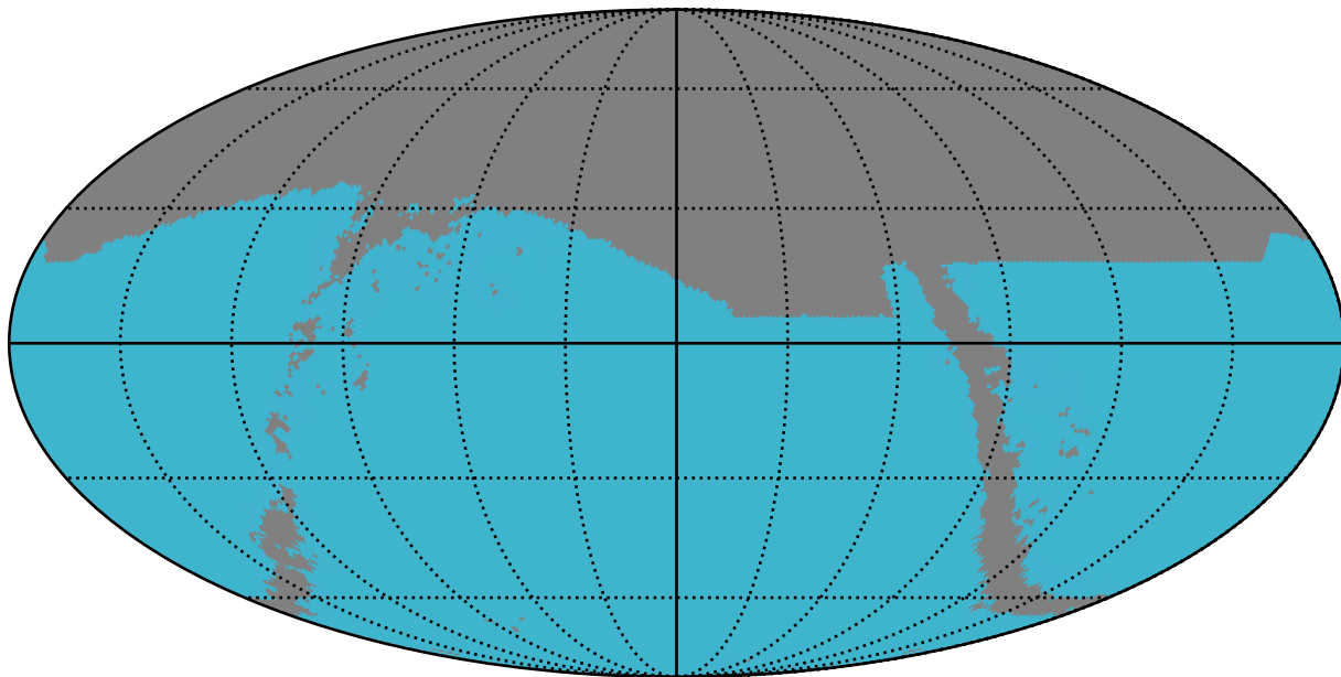
too_elab_r16_d3_ugrizy_v3.4_10yrs : SNSLMetric
