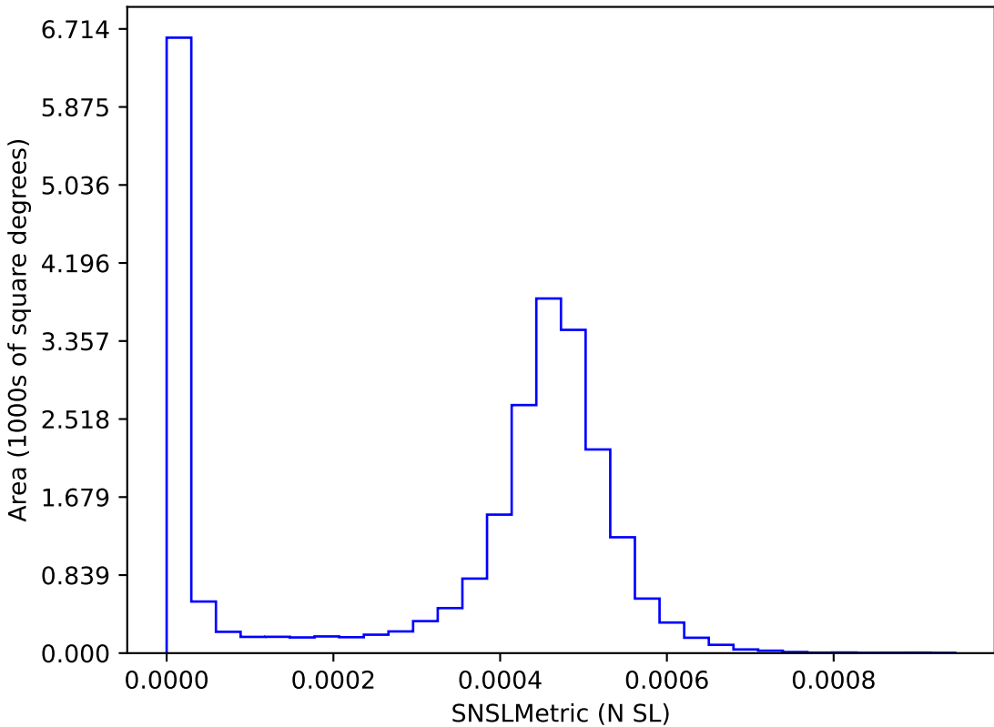
too_elab_r16_d3_ugrizy_v3.4_10yrs : SNSLMetric
