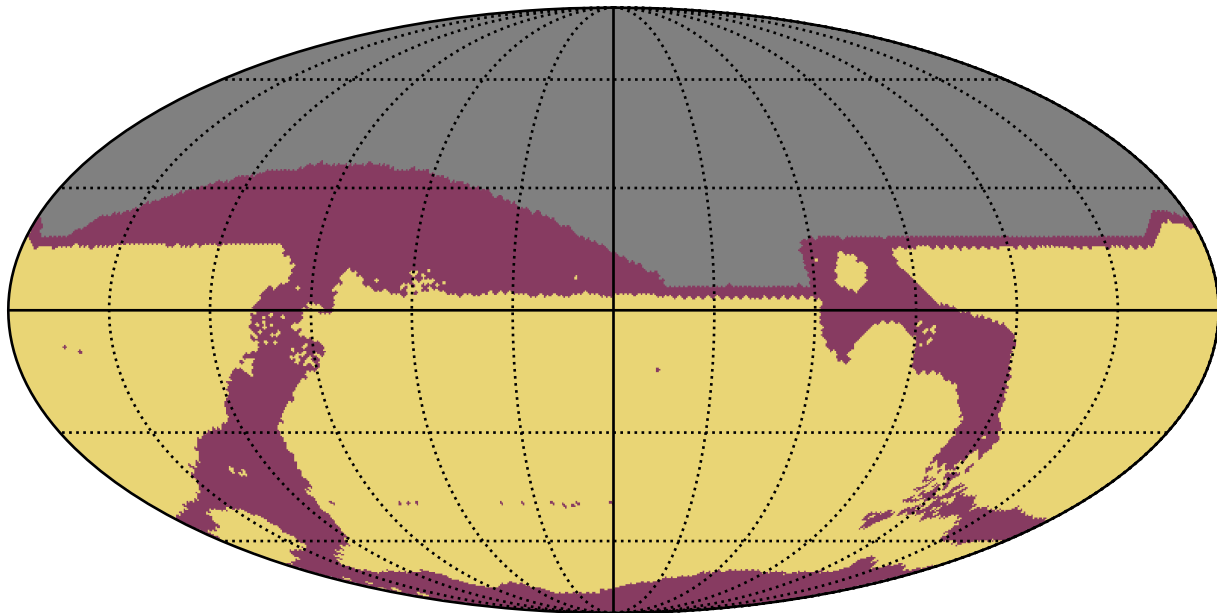
too_elab_r16_d3_ugrizy_v3.4_10yrs : RapidRevisits
