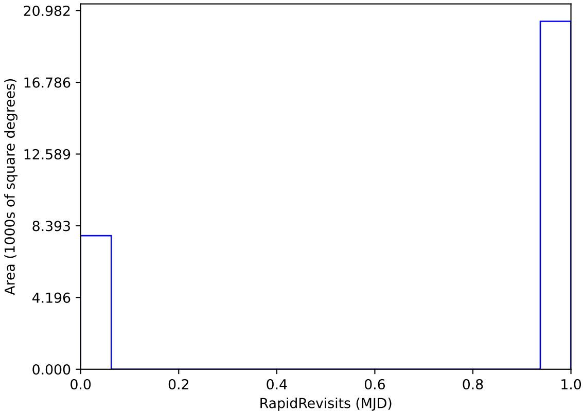
too_elab_r16_d3_ugrizy_v3.4_10yrs : RapidRevisits
