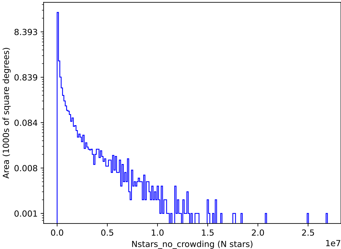
too_elab_r16_d3_ugrizy_v3.4_10yrs i: Nstars_no_crowding
