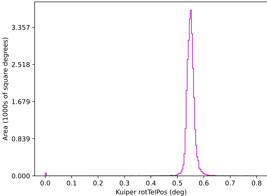
too_elab_r16_d3_ugrizy_v3.4_10yrs z: Kuiper rotTelPos
