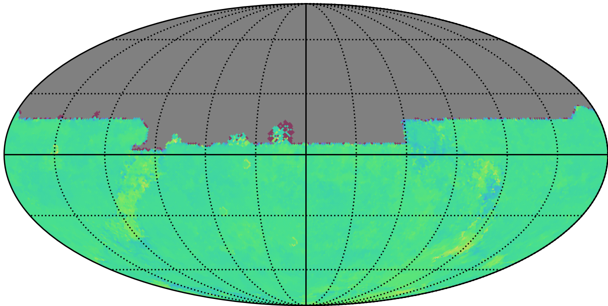
too_elab_r16_d3_ugrizy_v3.4_10yrs u: Kuiper rotTelPos
