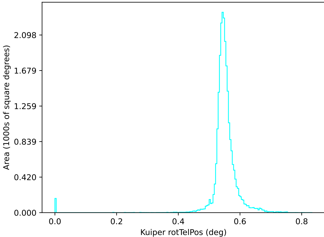
too_elab_r16_d3_ugrizy_v3.4_10yrs u: Kuiper rotTelPos
