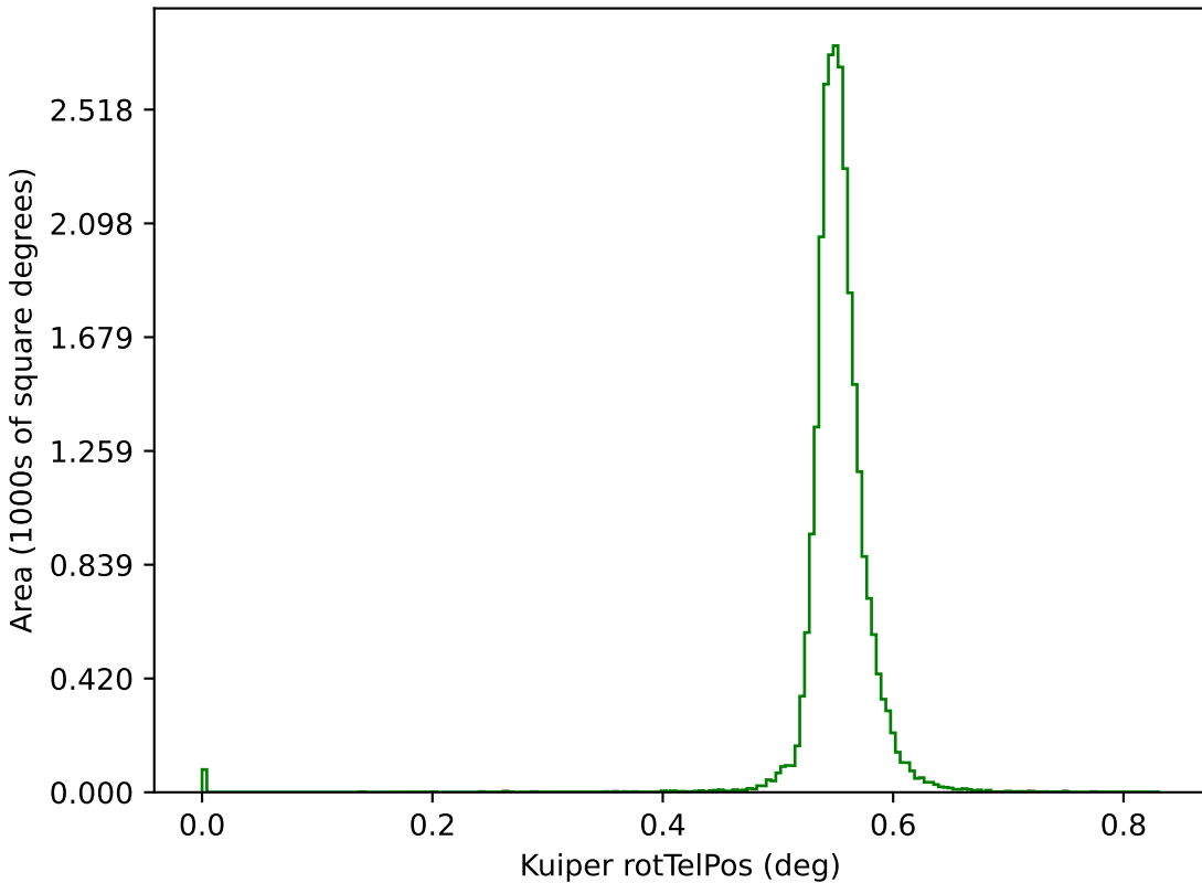
too_elab_r16_d3_ugrizy_v3.4_10yrs g: Kuiper rotTelPos
